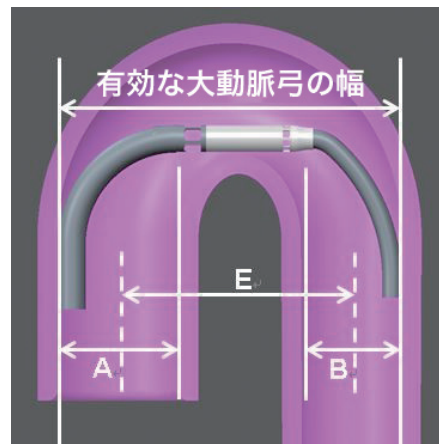
図7.3 屈曲の限界（大腿動脈からの挿入）
