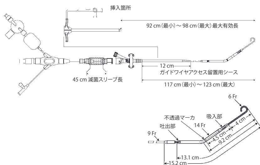
図7.2 IMPELLA CP SmartAssist カテーテル寸法
