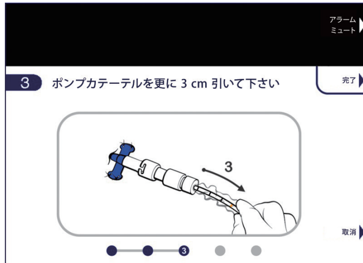
図5.9 カテーテルを更に 3 cm 引き戻す
