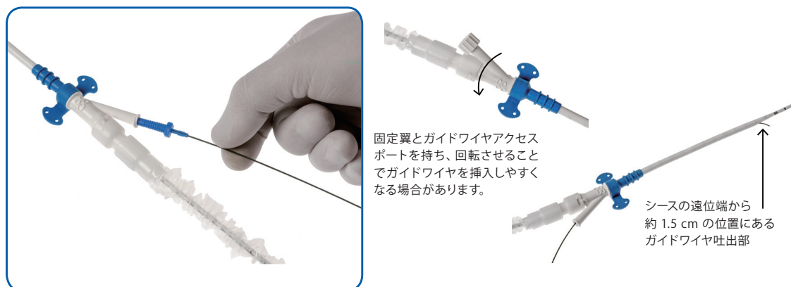
図4.34 インサータを用いてガイドワイヤを挿入
