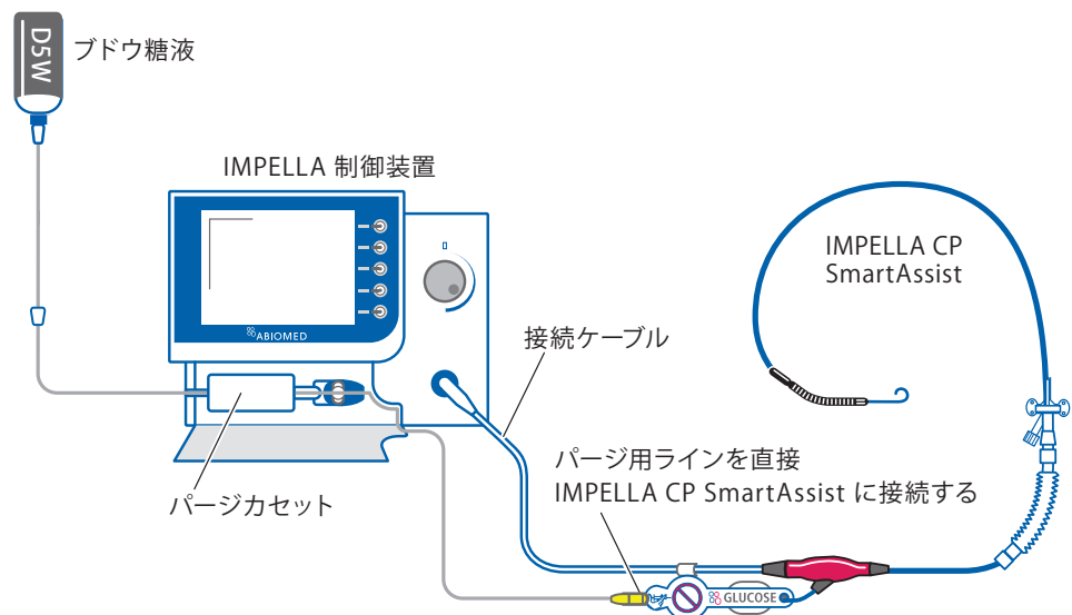
図2.2 IMPELLA 制御装置、IMPELLA CP SmartAssist、付属品、併用品の接続
