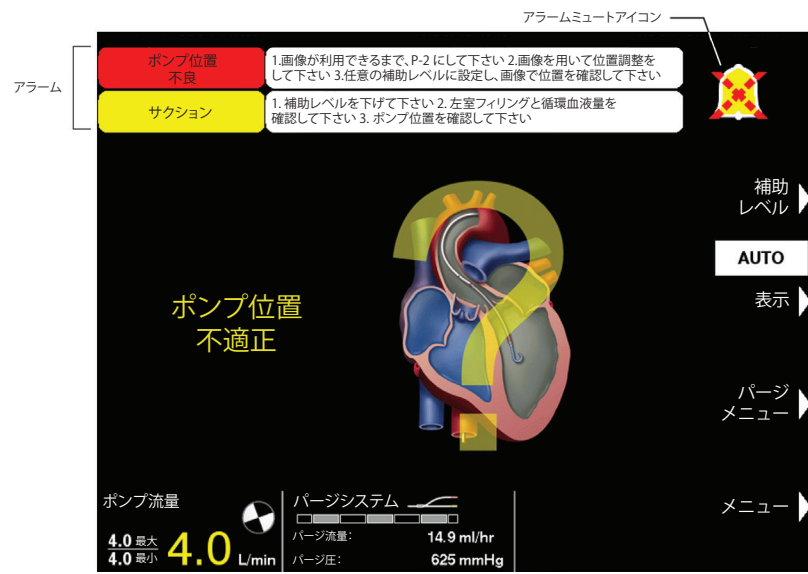
図6.1 アラーム表示
