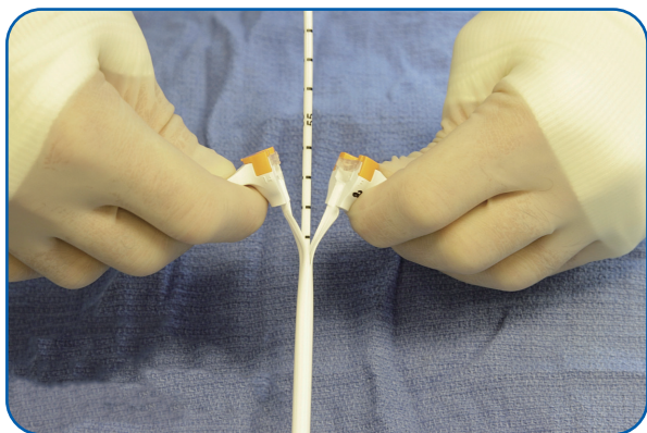
図4.29 ピールアウェイ式イントロデューサの抜去
