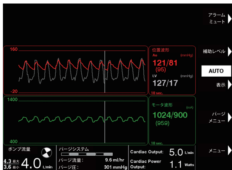
図5.5 適正な留置位置の IMPELLA CP SmartAssist
