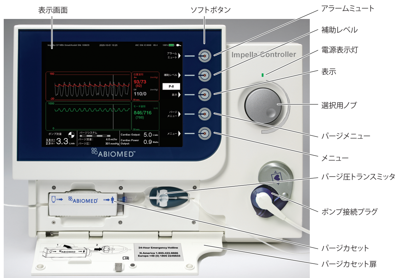
図3.1 IMPELLA 制御装置の特徴 – 前面図
